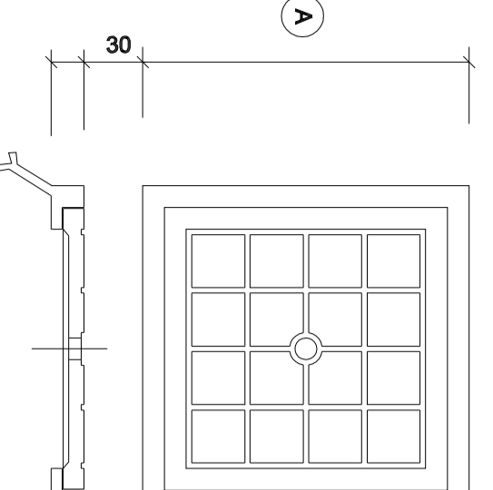
DETALLE DE TAPA COTAS EN CM
