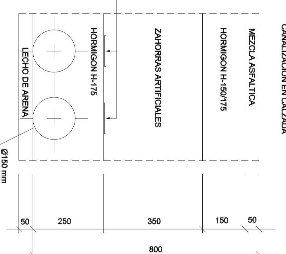
DETALLE DE CANALIZACIÓN COTAS EN CM
