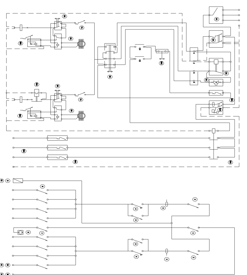
ESQUEMA UNIFILAR CENTRO DE MANDO
